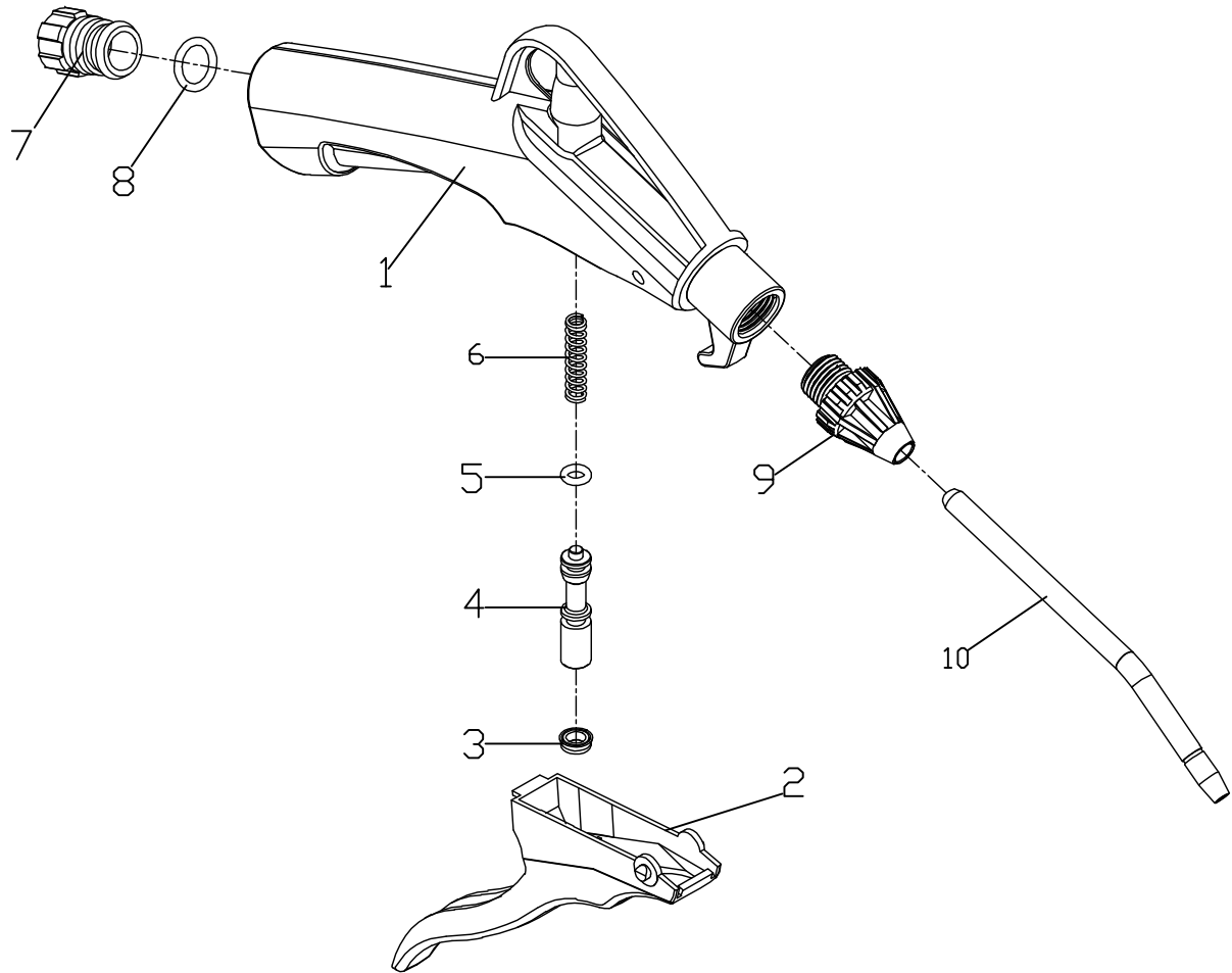
40B14 塑料吹尘枪爆炸图
