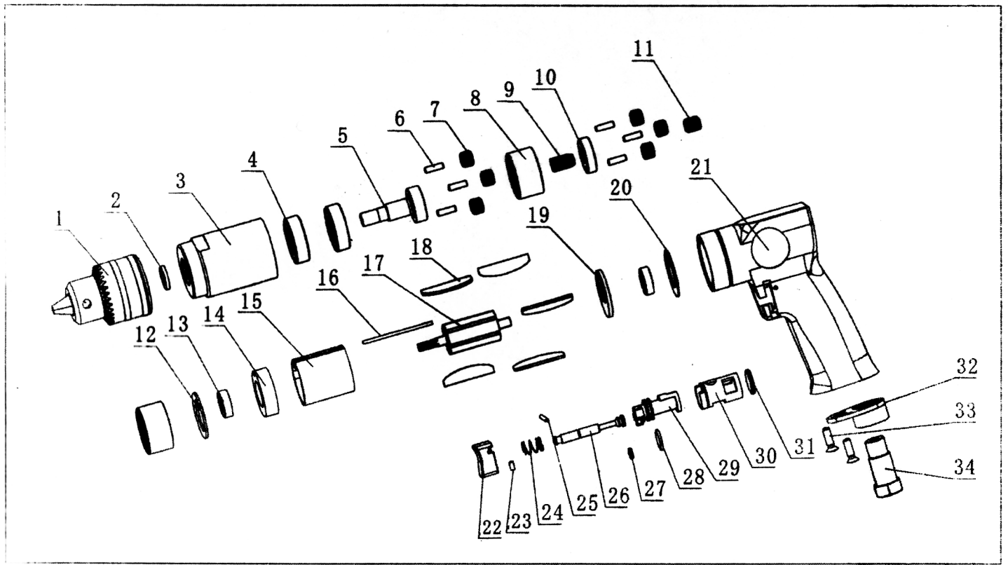
气钻爆炸图
